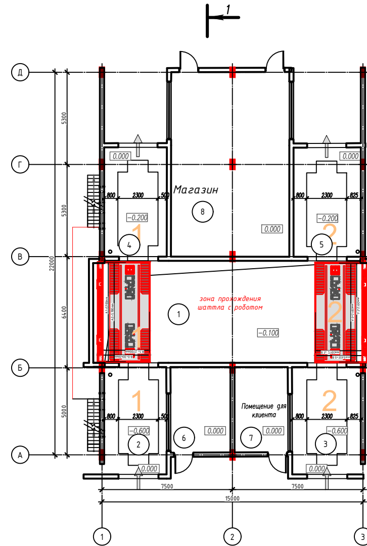
ПЛАН НА ЯРУСЕ ВЪЕЗДА
