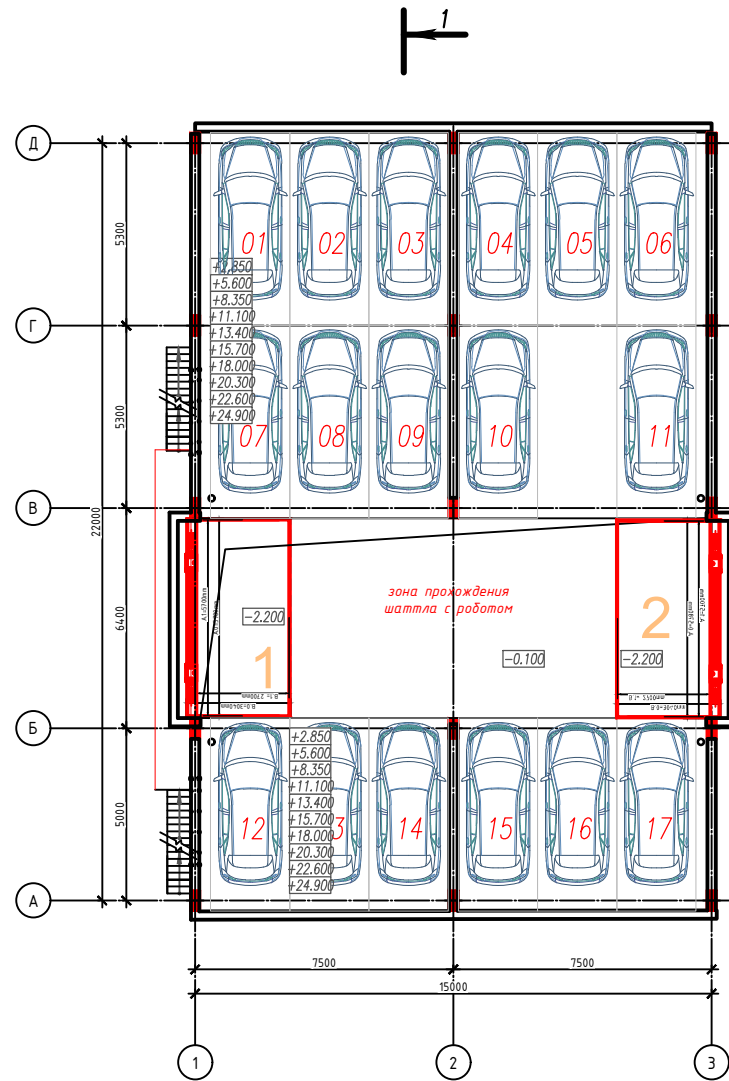
ТИПОВОЙ ЯРУС ХРАНЕНИЯ
