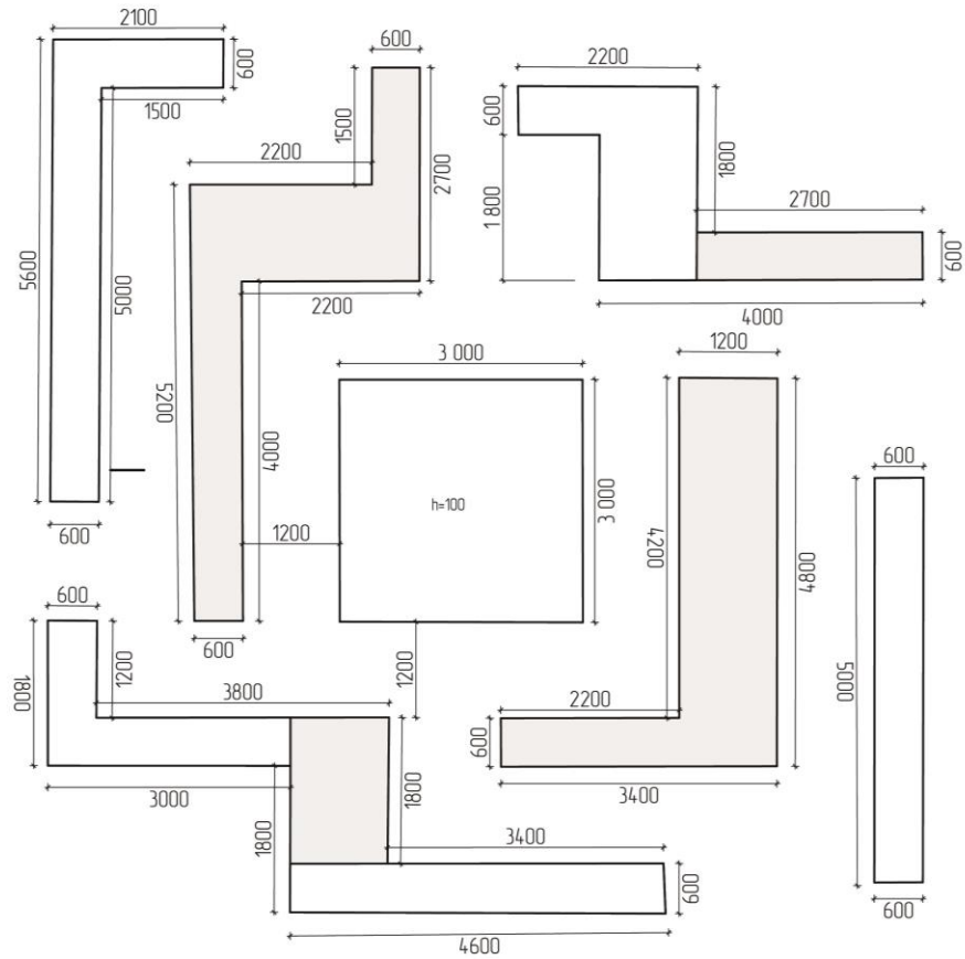
План бетонных оснований
