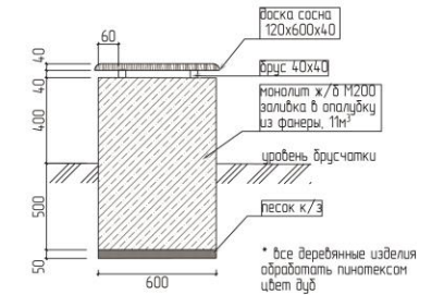
Разрез А-А
